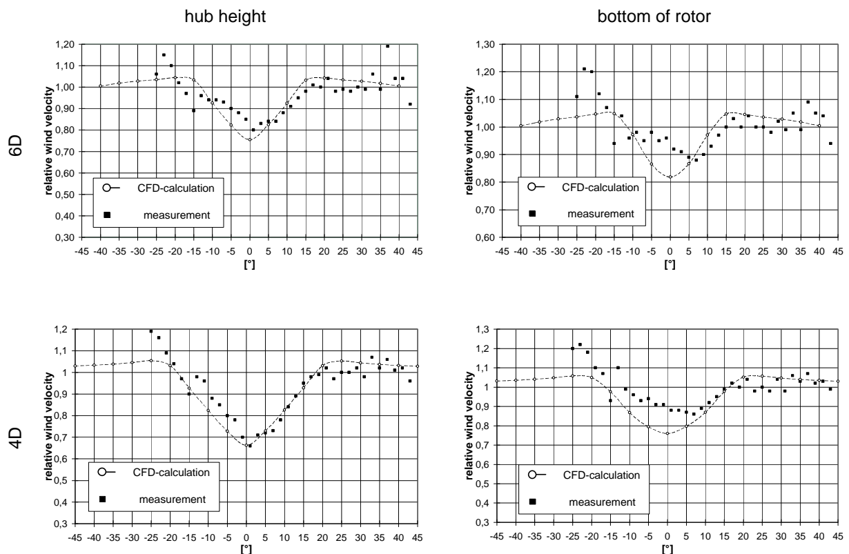
Abb. 2: Verhältnis von Windgeschwindigkeit zur Windgeschwindigkeit in der ungestörten Strömung. Die Gradangabe bezeichnet den Winkel zwischen der Windrichtung und der Achse Rotornabe-Messpunkt. (Messungen aus /4/).
