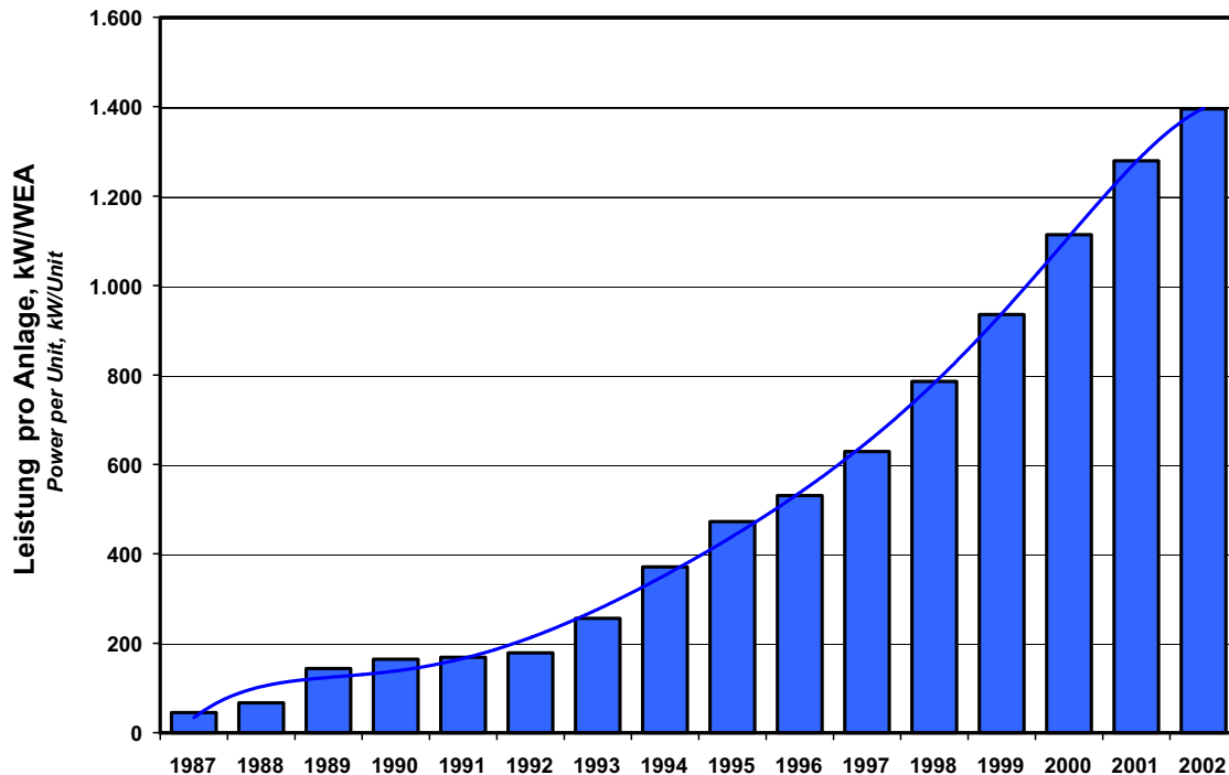
Abb. 5: Entwicklung der durchschnittlich installierten Leistung pro Windenergieanlage. Mit einer durchschnittlichen installierten Leistung im Jahr 2002 von 1.394,74 kW/Anlage liegt dieser Wert um ca. 9 % über dem Wert des Vergleichszeitraumes des Vorjahres. Fig. 5: Development of the average installed power per unit. The introduction of the megawatt-class leads to an increase of the average installed capacity per WT. The value of 1,394.74 kW/unit in 2002 is about 9 percent higher than for the same period of 2001.
