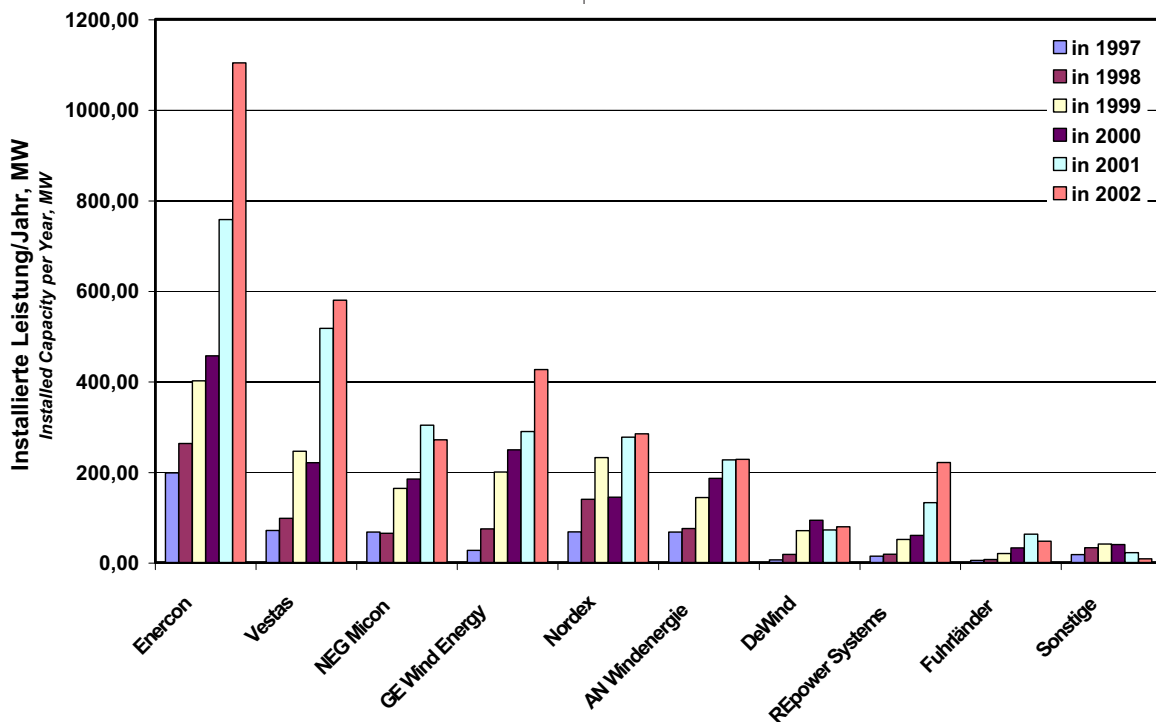
Abb. 7: Entwicklung der jährlichen installierten Leistung der in Abb. 8 und 9 genannten Hersteller in Deutschland seit 1997. Fig. 7: Development of the yearly installed power of the manufacturers named in Fig. 8 and 9 in Germany since 1997.
